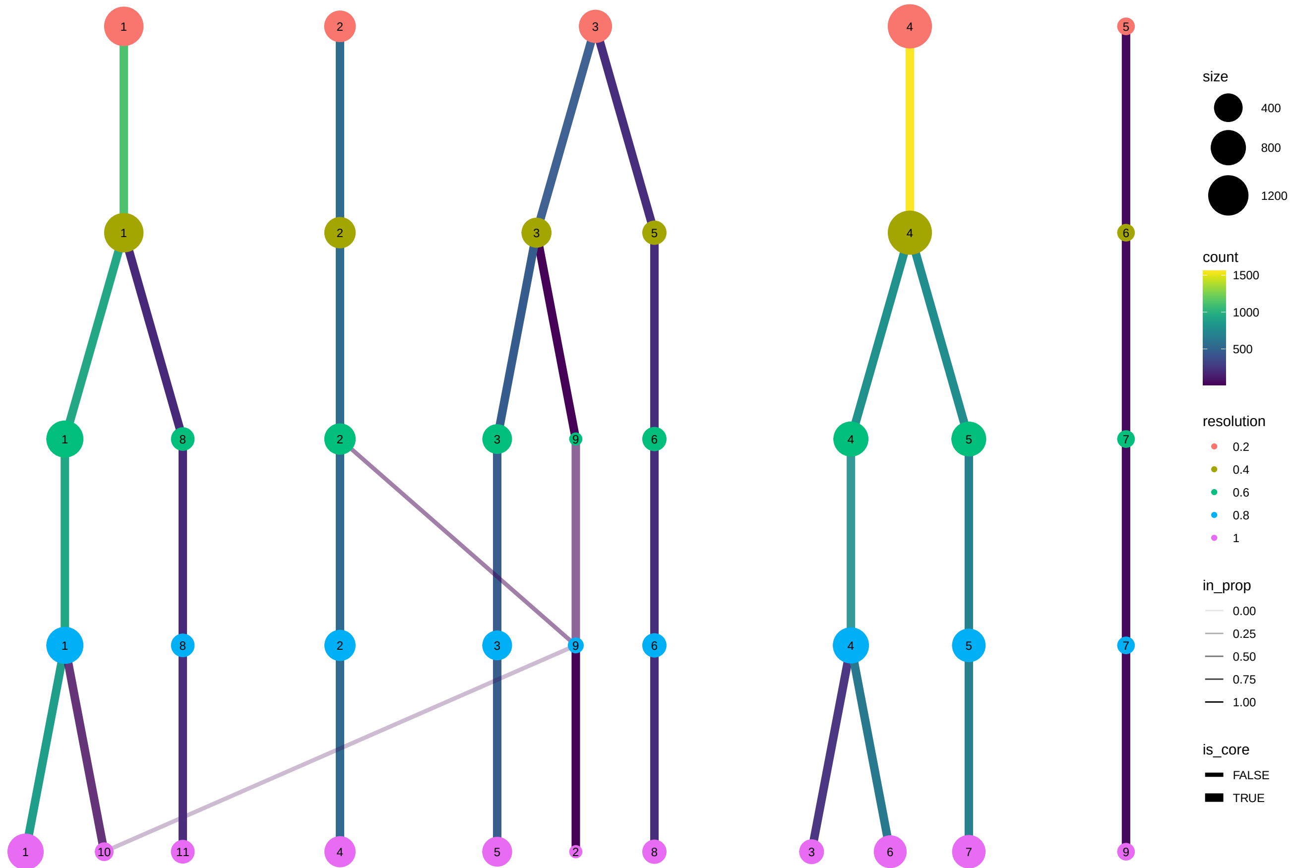
cluster_int_graph_louvain
